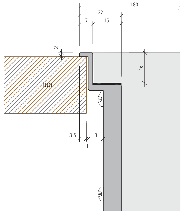
sezione del bordo / frame section
