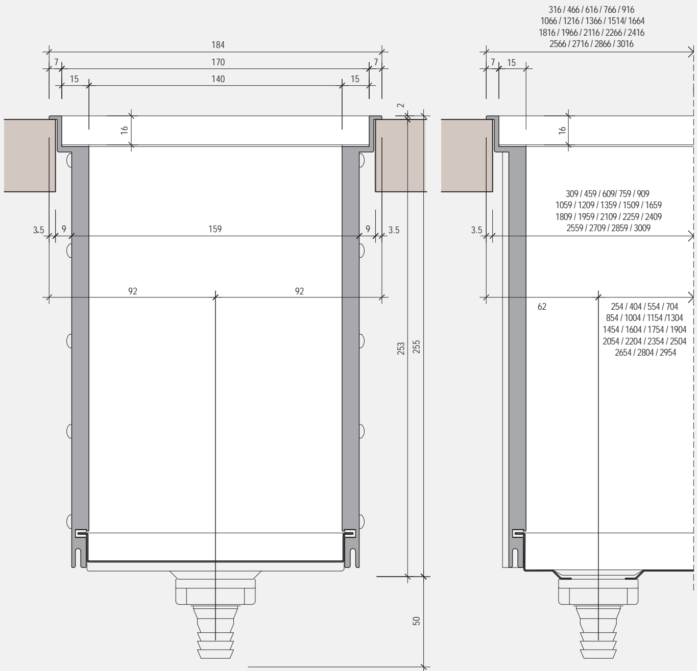
AA - sezione trasversale / AA - cross section
